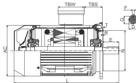
IM B5 - D Flange
